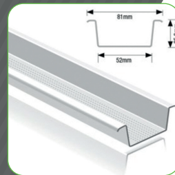
MF5 Tophat
