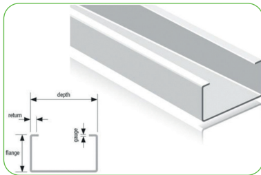
SFS Stud
