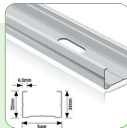
Acoustic Stud
